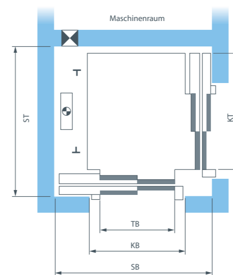
Schachtabmessung für Übereck-Zuladung auf Anfrage
